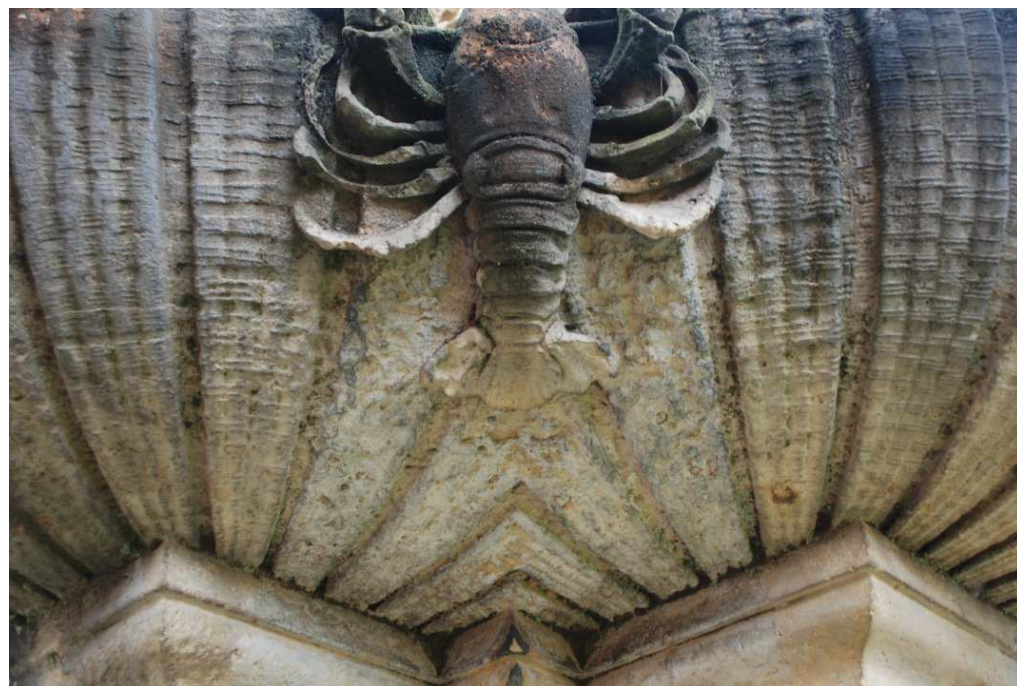
Horní mísa s chrličí. Výkvěty solí na spodní straně mísy.
